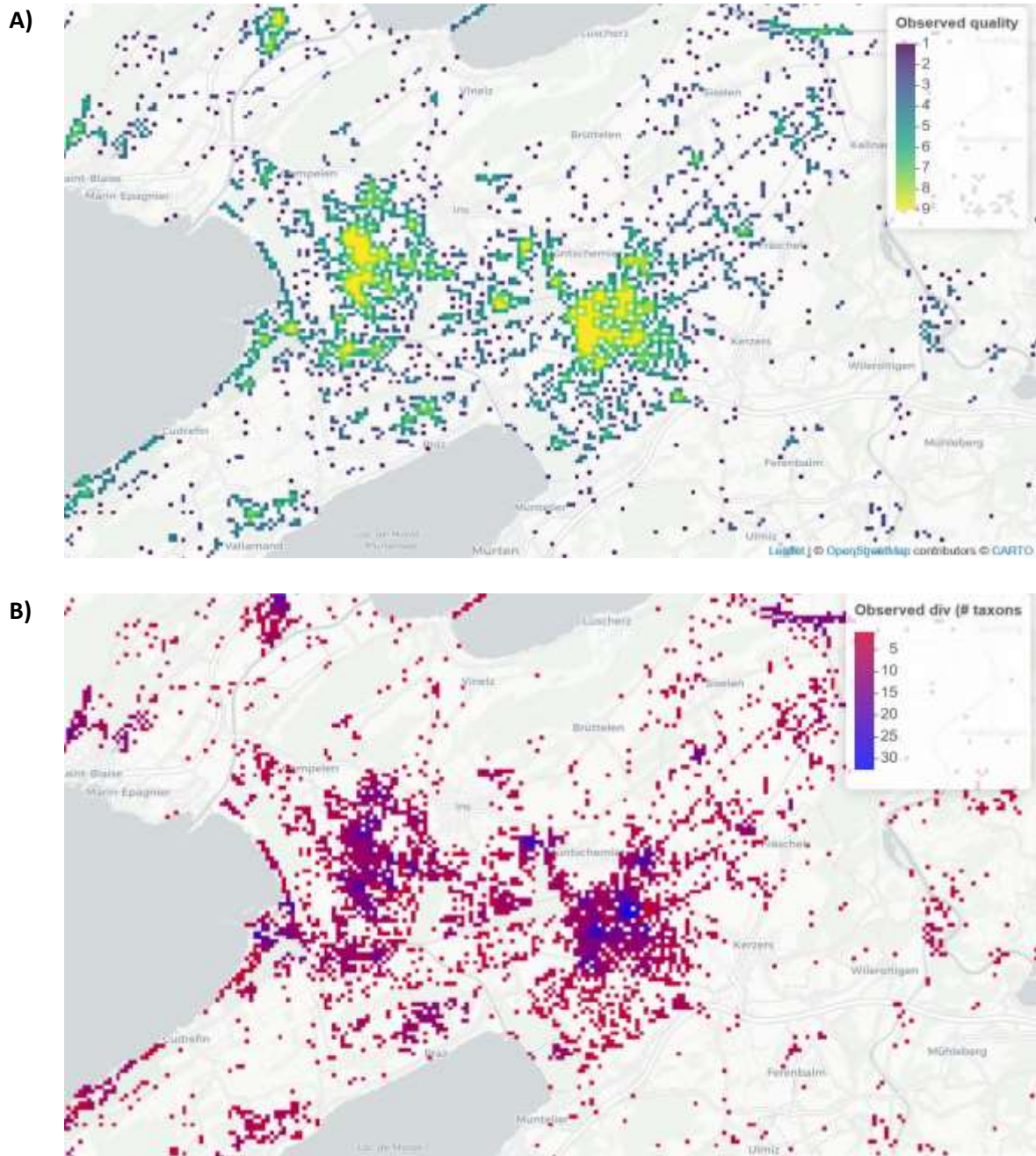
Figure 4: Exemples de cartes représentant la qualité observée des guildes mobiles (guilde 25). Les hectares colorés indiquent la présence d'espèces indicatrices dans le paysage environnant pour la guildie considérée. A) Qualité paysagère observée : plus la couleur d'un hectare tend vers le jaune, plus le nombre d'hectares dans la fenêtre paysagère abritant des espèces indicatrices (au minimum une observation par hectare) est important. B) Nombre d'espèces indicatrices observées : plus la couleur d'un hectare tend vers le bleu, plus le nombre d'espèces annoncées dans la fenêtre paysagère est important. Les habitats inappropriés à chaque guildie ont été exclus (ici : agglomérations, forêts et surfaces d'eaux ouvertes), de telle sorte que des observations d'espèces indicatrices hors espace-guildie n'apparaissent pas sur la carte. Exactement les mêmes hectares sont mis en évidence par les deux variables « qualité paysagère observée » et « nombre d'espèces indicatrices observées » dans la fenêtre ; ceux-ci affichent uniquement une valeur différente et constituent des informations complémentaires pour la planification et la mise en œuvre.
