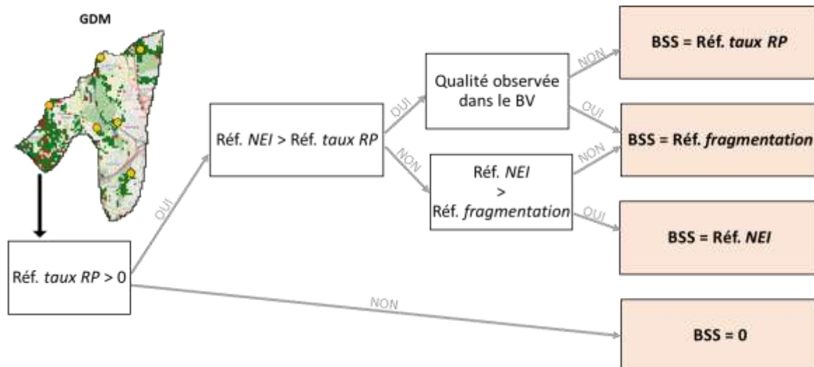
Figure 20: Représentation synthétique de l'approche pour estimer le besoin en surfaces supplémentaires (BSS) pour chaque guild. Un modèle de distribution environnementale (GDM) est calibré et projeté dans l'espace-guilde afin de délimiter une distribution potentielle de la qualité pour la guild. Pour chaque bassin versant, trois valeurs de BSS sont calculées, selon trois états de références : premièrement, un état de référence pour le taux de remplissage de la qualité potentielle (Réf. Taux RP), deuxièmement, un état de référence pour le nombre d'espèces indicatrices (Réf. taux NEI) et troisièmement, un état de référence pour limiter la fragmentation de la guild (Réf. fragmentation). L'arbre de décisions ci-dessus permet ensuite de sélectionner un de ces trois états de référence pour fixer une valeur de BSS finale.
