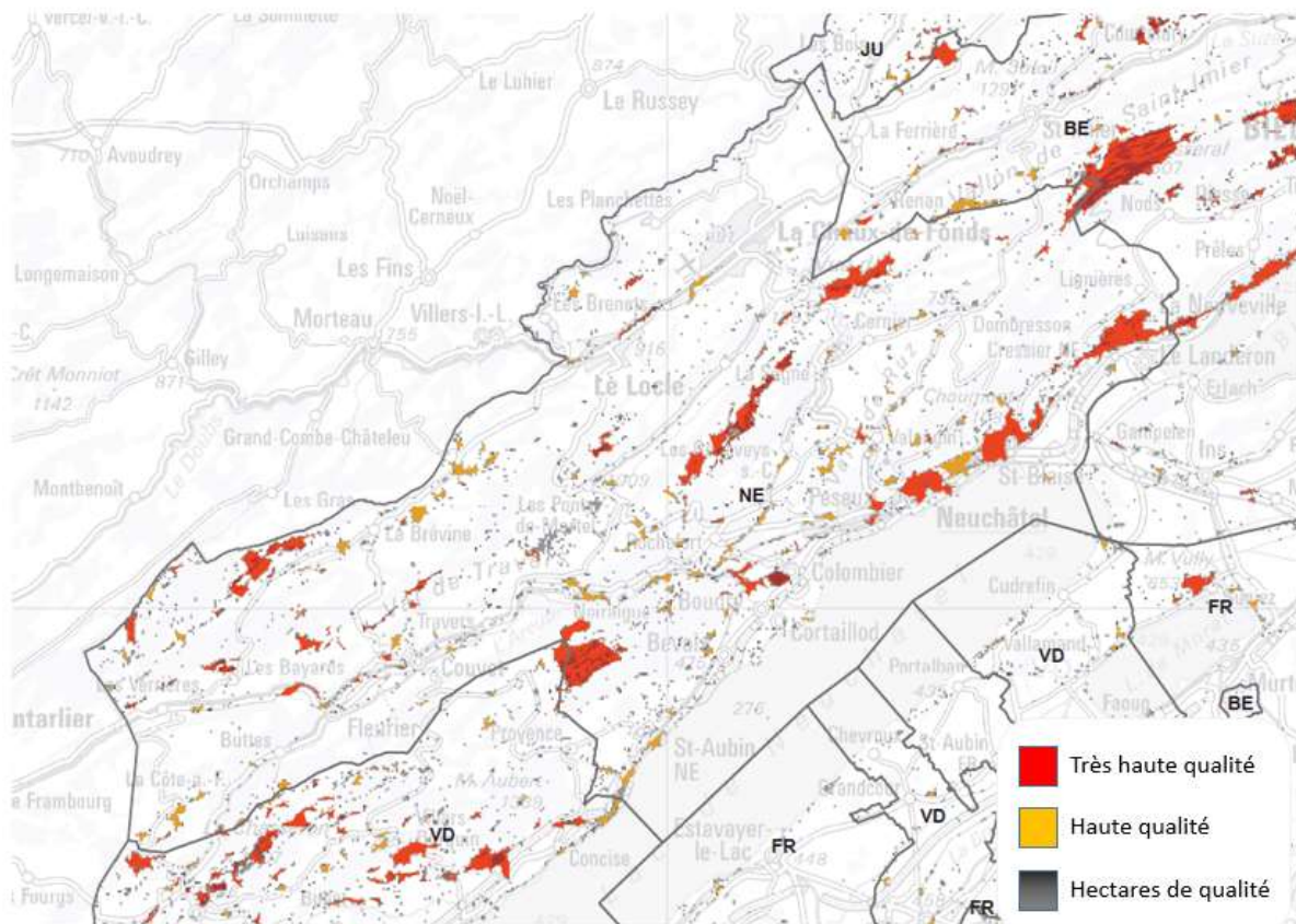
Figure 11 : Exemple de polygones d'agrégation de très haute qualité (rouge) et de haute qualité observée (jaune) pour la guild 14 (prairies et pâturage secs ; prés gras riches en espèces) dans le canton de Neuchâtel. Les hectares de qualité observée sont également représentés (en noir).
