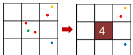
Figure 3 : Mode de fonctionnement de la fenêtre mobile pour modéliser la qualité observée des guildes mobiles à l'échelle du paysage. A) Qualité paysagère observée. Contrairement aux guildes sessiles, une valeur de 1 a été attribuée à toutes les espèces de vertébrés indicatrices, ce qui signifie que la présence d'une seule espèce remplissant les critères du chapitre 2.2 suffit pour qu'un hectare soit considéré comme de qualité observée. B) Nombre d'espèces indicatrices observées. Cette deuxième variable a été retenue comme indicateur complémentaire à la qualité paysagère observée, cette dernière n'intégrant aucune information sur la diversité des espèces rencontrées.
