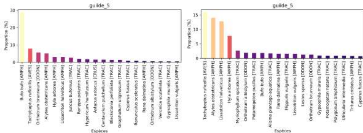
Figure 12 : Graphiques montrant la contribution des 20 premières espèces dans l'analyse pour la guilde 5. Sur l'image de gauche avec Bufo bufo , qui est une espèce à large répartition au niveau national et à droite après suppression de celle-ci.
