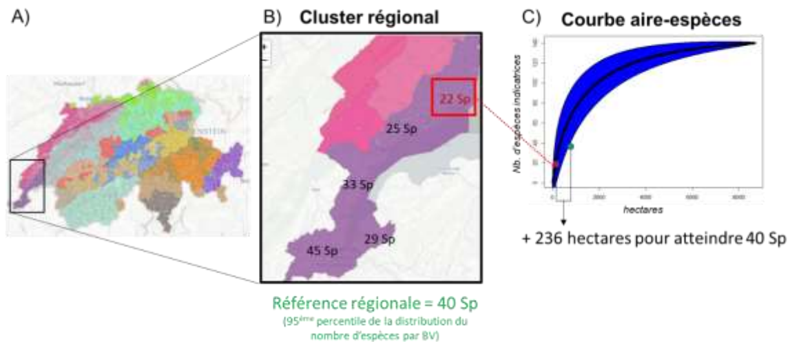
Figure 16 : Calcul de la première référence pour l'estimation des BSS : nombre d'espèces indicatrices observées par bassin versant. A) Pour chaque guild, les bassins versants (BV) ont été groupés en clusters régionaux (distingués par leurs couleurs) en fonction de leurs similarités biogéographiques, topographiques et environnementales. B) Le nombre d'espèces indicatrices présentes dans chaque BV est connu. Au sein de chaque cluster, le 95 ème percentile des nombres d'espèces par BV est utilisé comme état de référence pour tous les BV appartenant au cluster considéré. C) La distribution des espèces indicatrices est utilisée pour calibrer une courbe aire-espèces au sein de chaque cluster régional. Pour chaque BV, le nombre d'hectares à ajouter (en fonction du nombre d'espèces) correspond à la différence entre le nombre d'hectares estimés pour l'état de référence (point vert) et le nombre d'hectares de qualité observée au sein du BV (point rouge). Sp = espèces.
